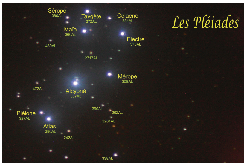
Noms et distances des étoiles de l'amas des Pléiades visibles à l'œil nu et magnifiques dans des jumelles.
